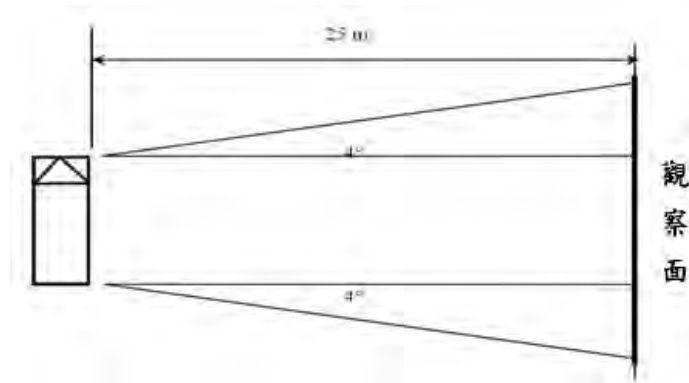
車輛側方反光標識可視性示意圖
