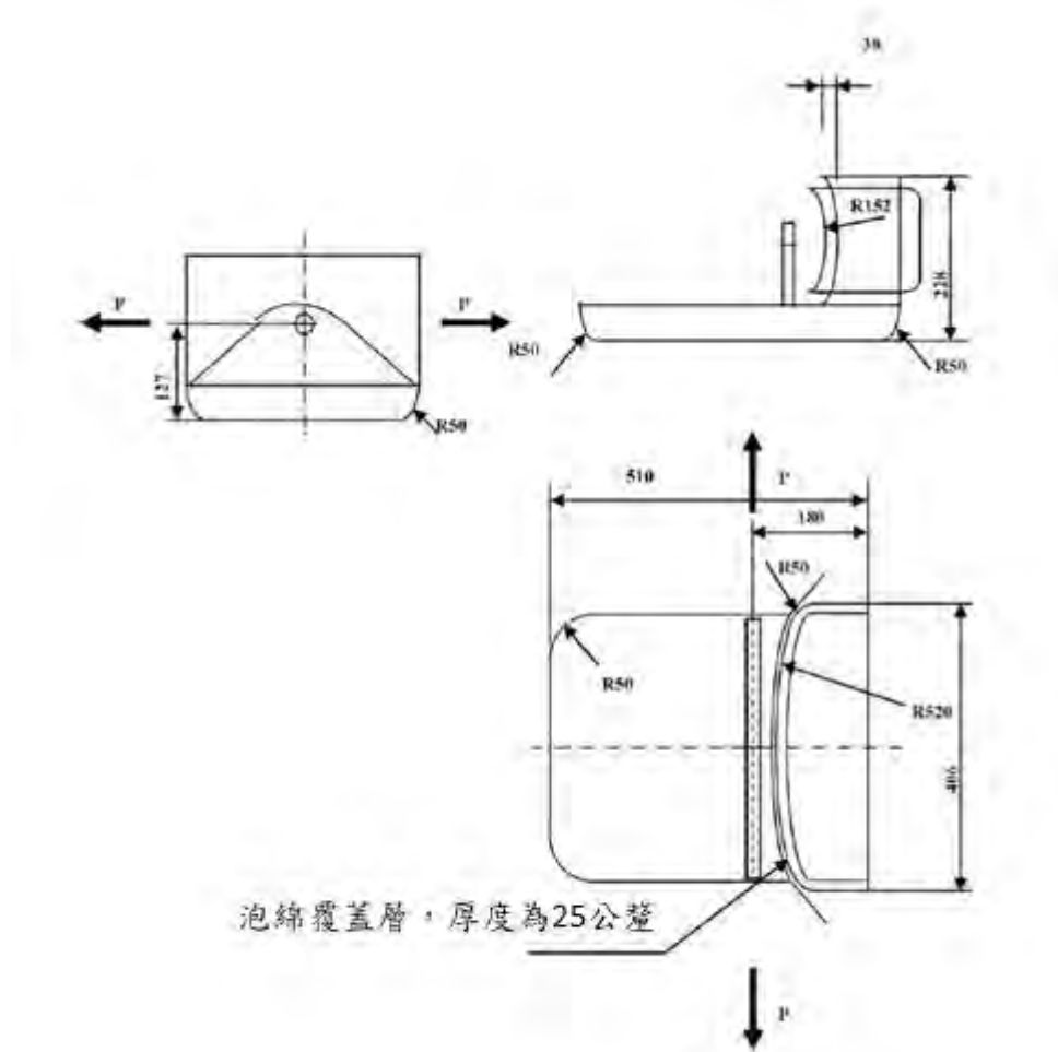
圖二十九：拉力裝置
