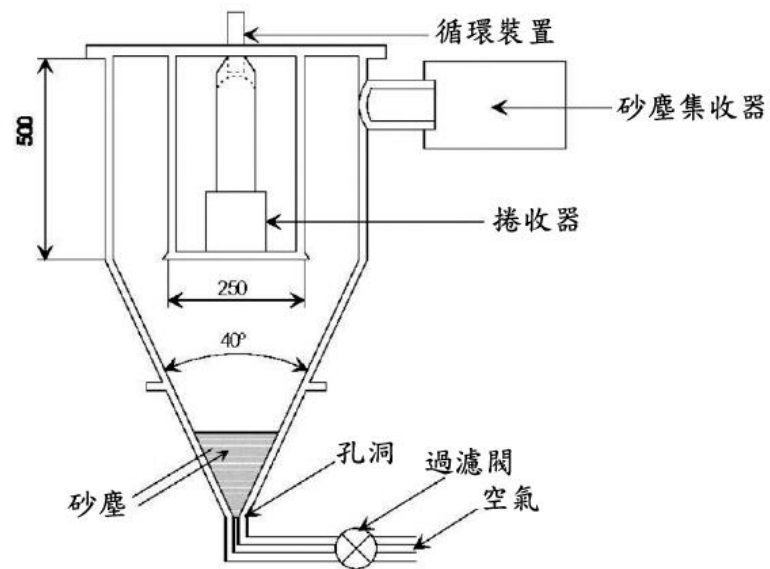
圖七：耐塵性試驗儀器示意圖
