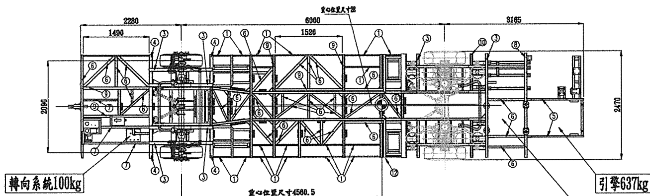
底盤五視、骨架資料及物件重量位置示意圖
