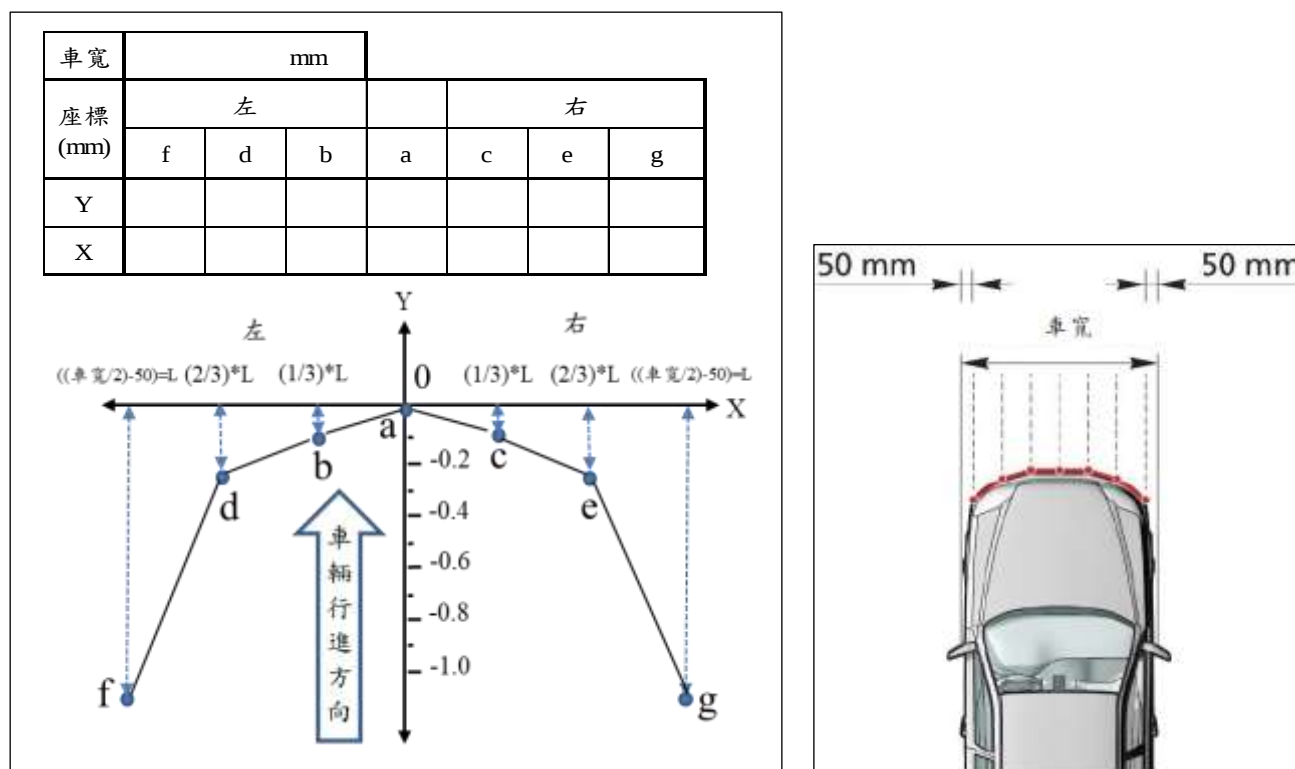
受驗車輛前保桿輪廓示意圖
