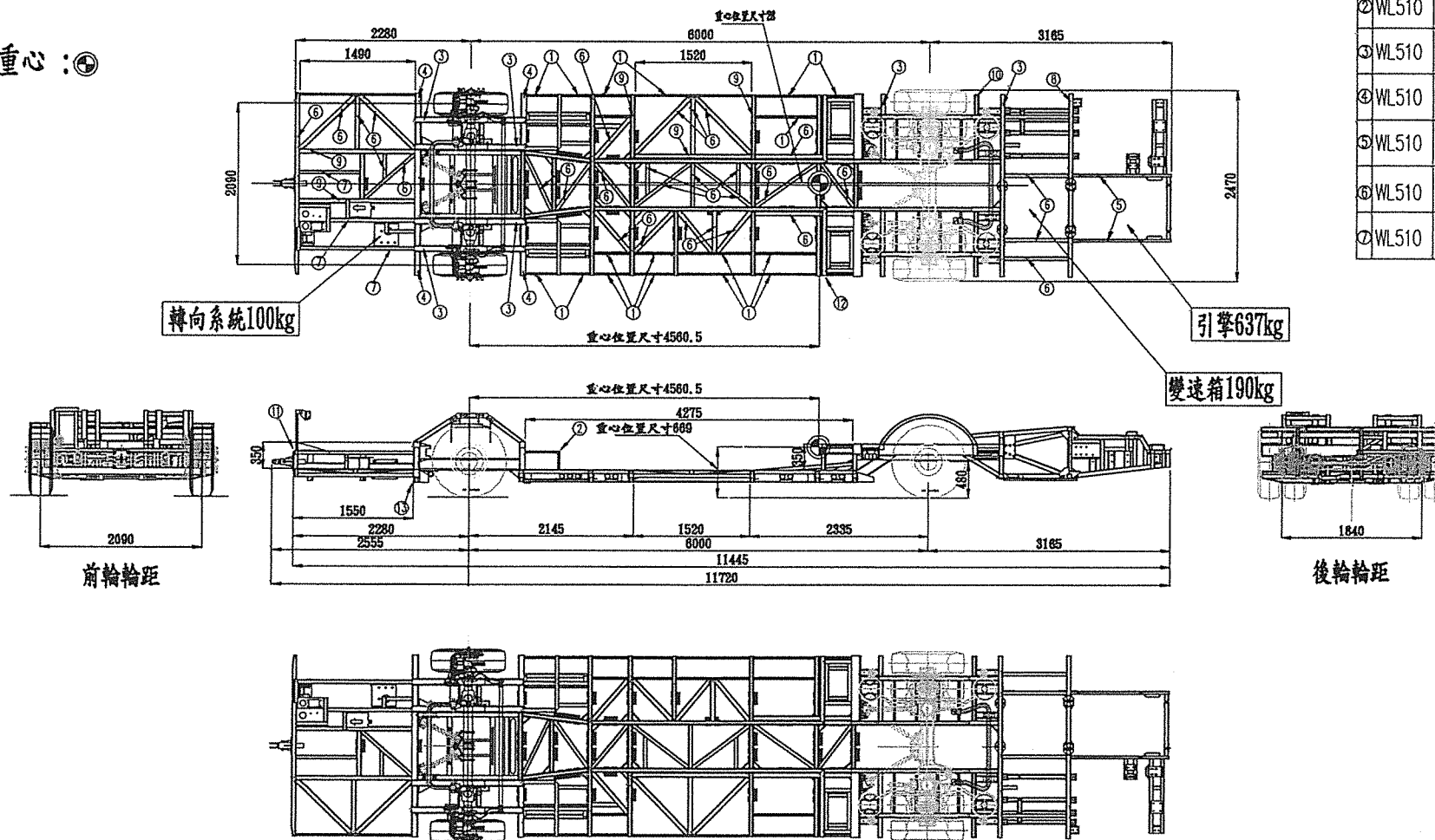
底盤五視、骨架資料及物件重量位置示意圖
