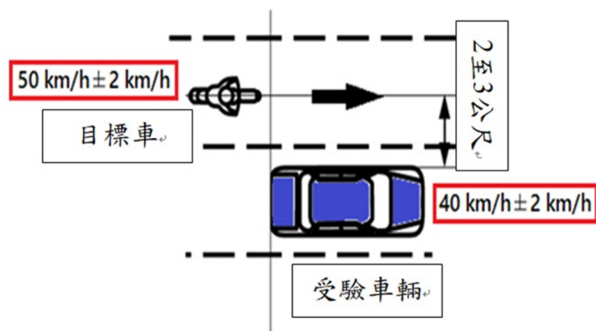
圖 4：目標車超越受驗車輛之車速示意圖
