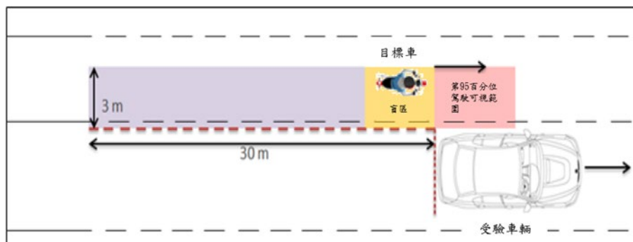
圖 7：提供駕駛盲點警示
