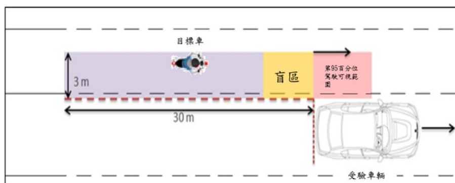
圖 6：非必須提供駕駛盲點警示
