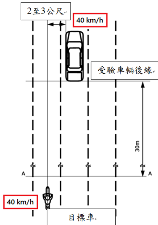
圖 3：目標車以穩定速度進入 30 公尺區域
