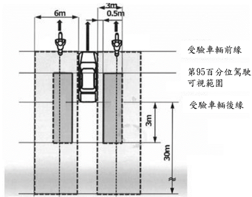
圖 14：盲點偵測區域
