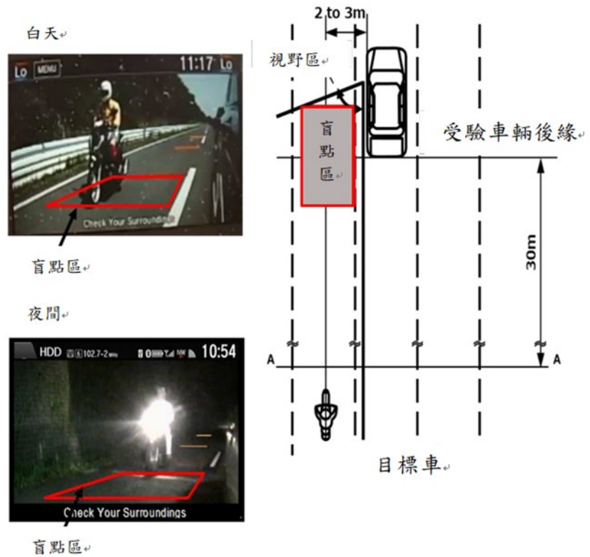
圖 17：盲點視覺系統之盲點區即時影像 備註：夜間試驗時，機車應開啟頭燈。
