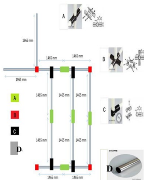
圖 2：盲點偵測涵蓋區域裝配架
