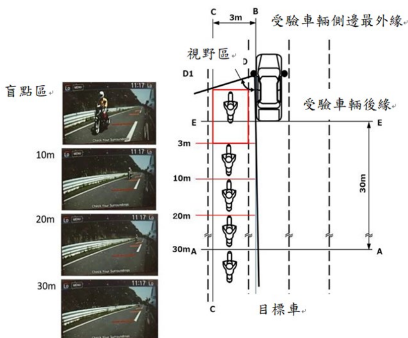
圖 16：功能確認與得分
