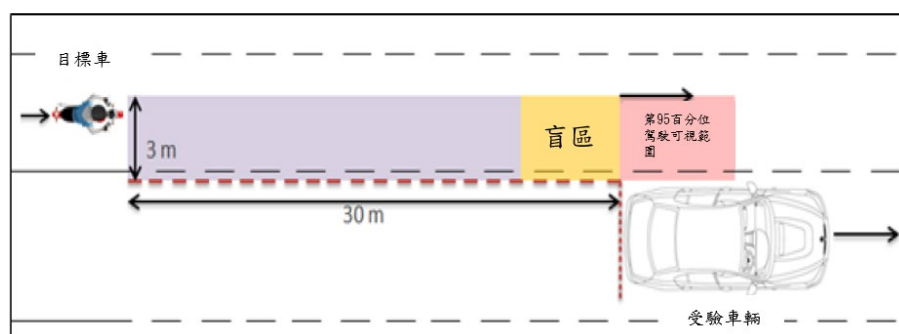
圖 5：不應提供駕駛盲點警示
