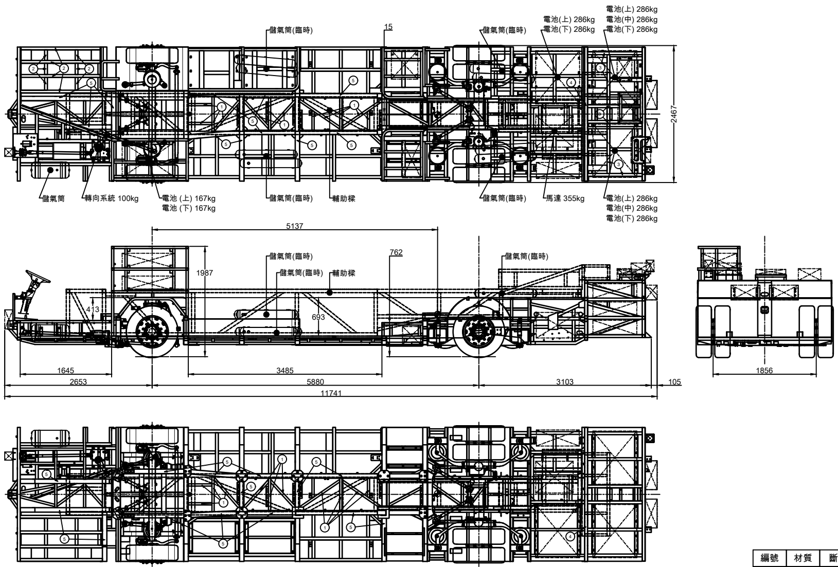
底盤五視、骨架資料及物件重量位置示意圖
